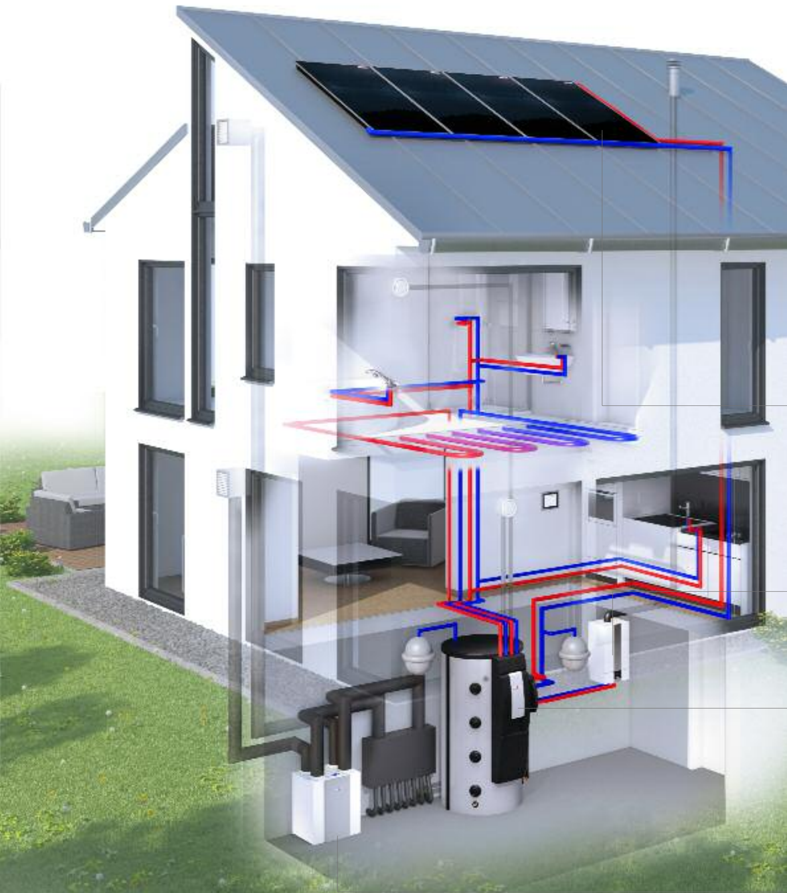
Esempio di sistema a condensazione con impianto solare e ventilazione meccanica
