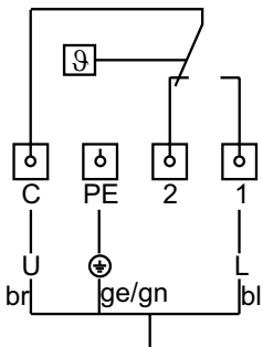
Câbles de raccordement du chauffe-eau
